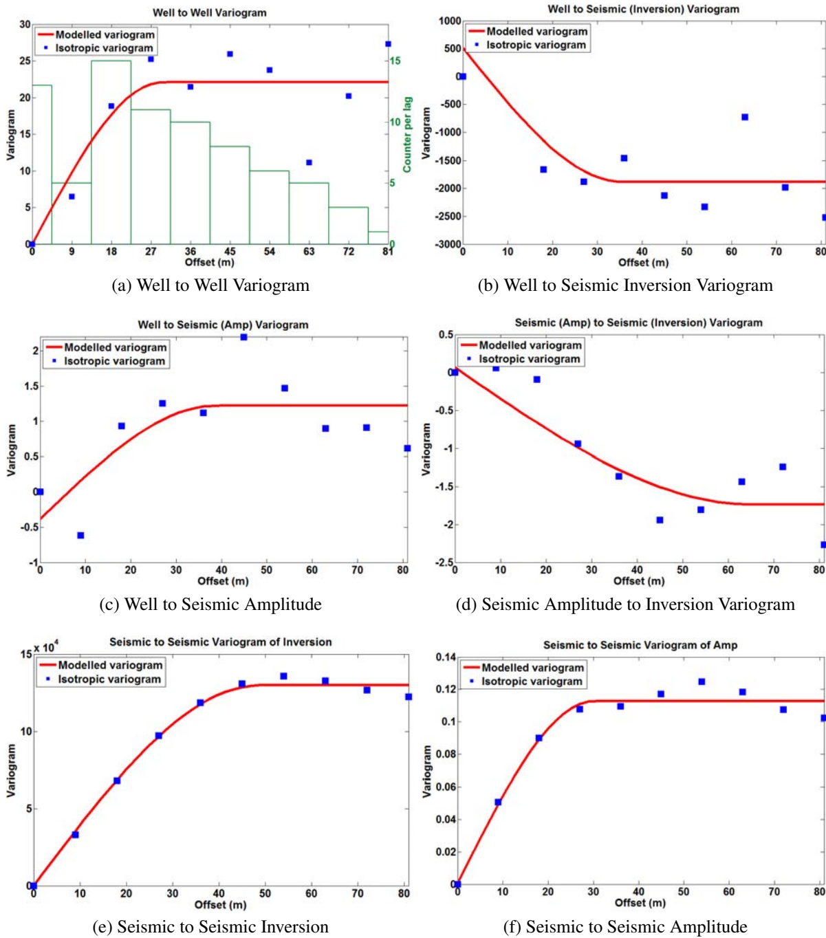
FIG. 5: Variograms
