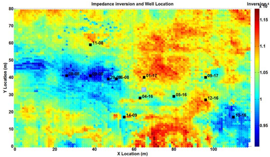
FIG. 3: Inversion slice
